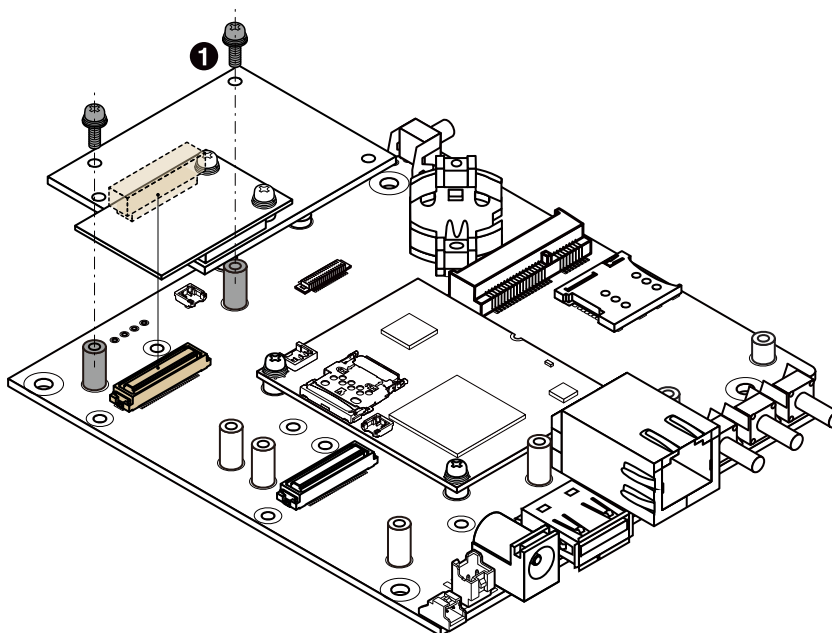
図 18.27 RS232C アドオンモジュールを CON2 に接続
