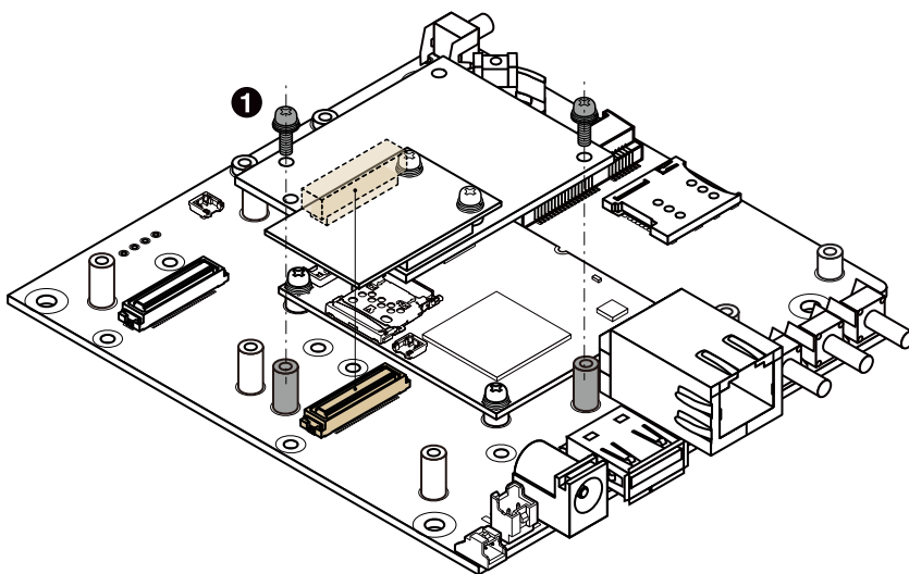
図 18.25 RS232C アドオンモジュールを CON1 に接続
