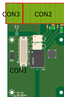
図 18.20 絶縁 IO アドオンモジュール インターフェースレイアウト
