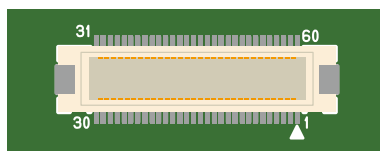
図 20.5 ベースボードとの接続コネクタのピン配置
