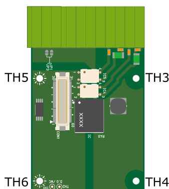
図 18.21 絶縁 IO アドオンモジュールの固定穴
