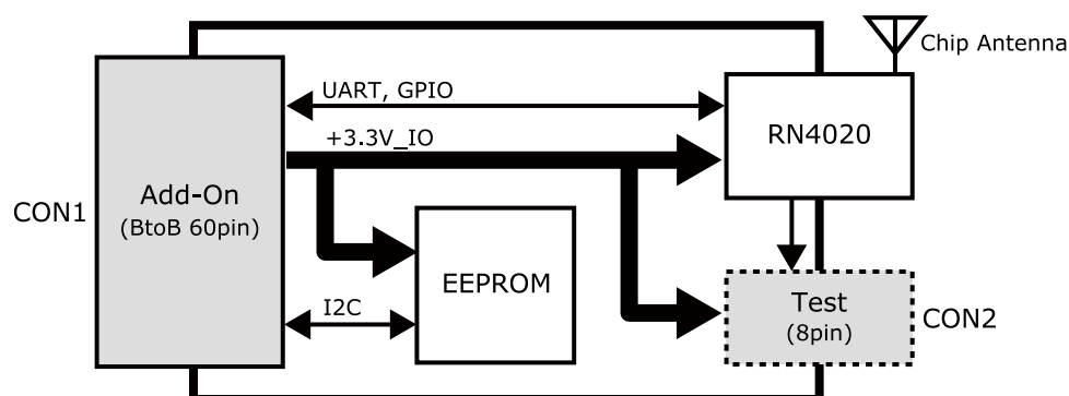
図 18.10 BLE アドオンモジュール ブロック図
