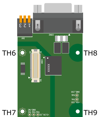
図 18.6 RS485 アドオンモジュールの固定穴
