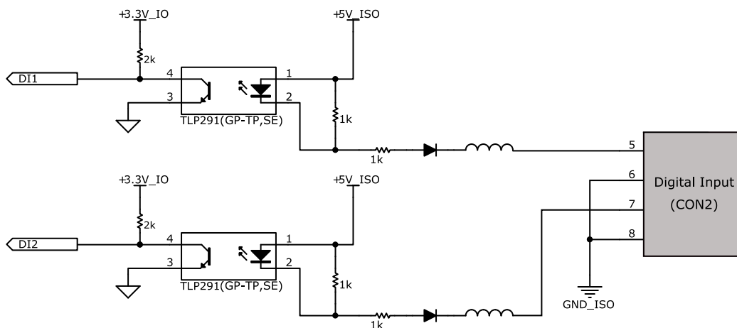
図 18.22 CON2 入力回路
