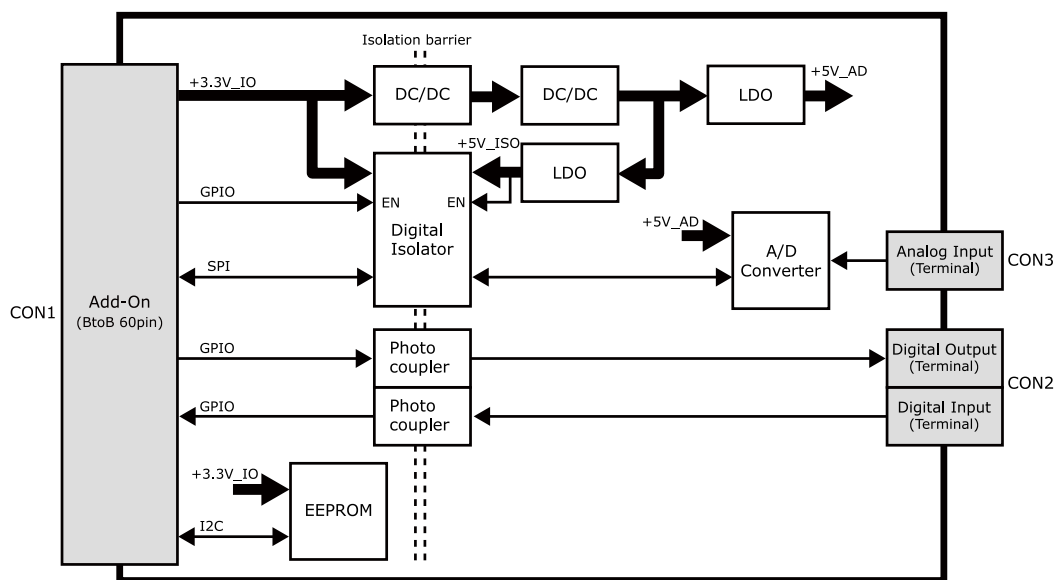
図 18.19 絶縁 IO アドオンモジュール ブロック図
