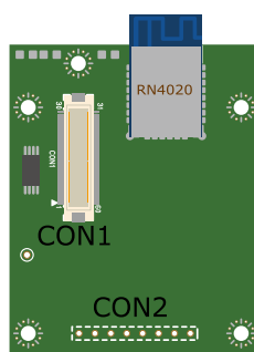
図 18.11 BLE アドオンモジュール インターフェースレイアウト
