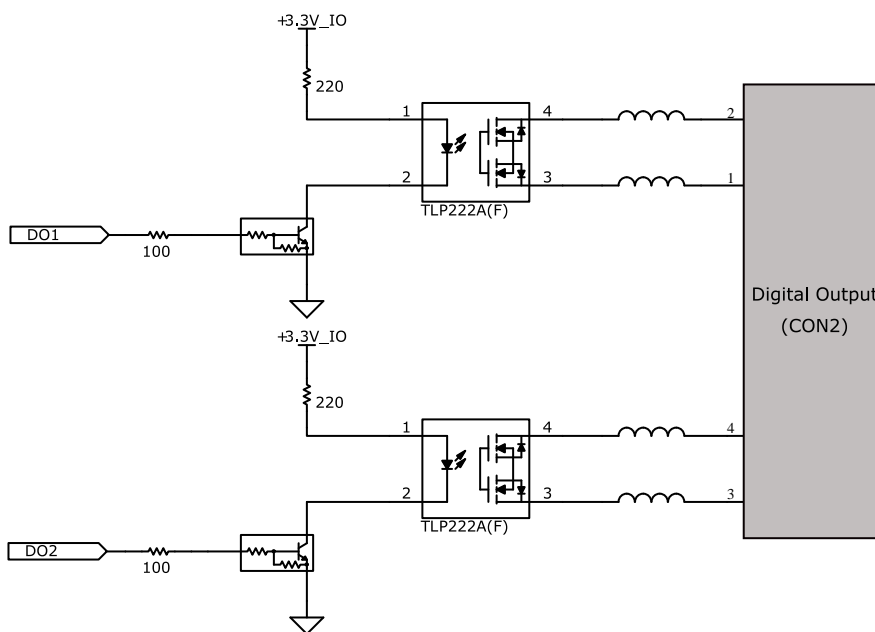
図 18.23 CON2 出力回路
