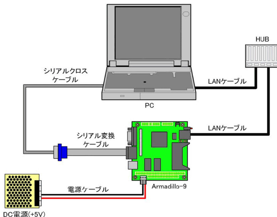
図 3.2 接続図
