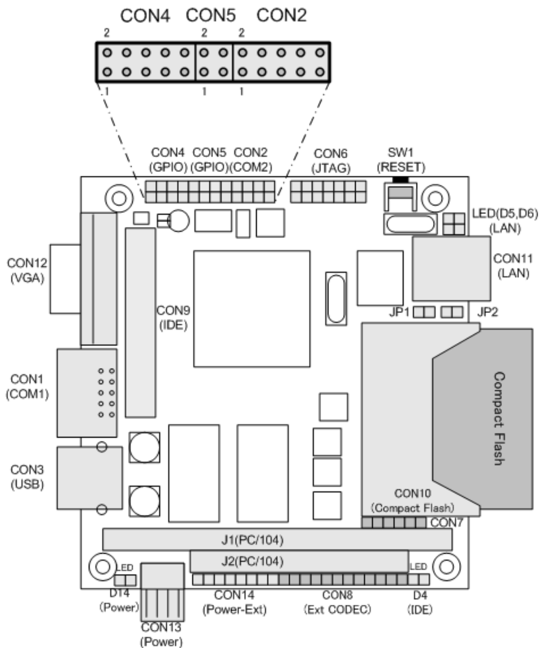
図 3.1 見取り図
