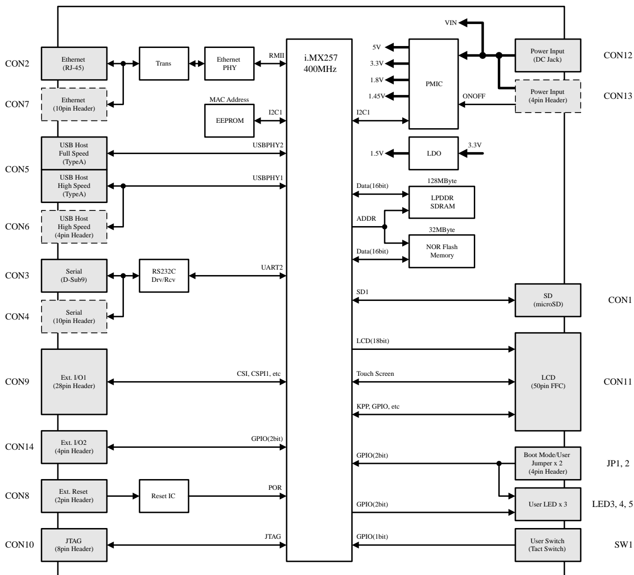
図 2.1 Armadillo-440 ブロック図
