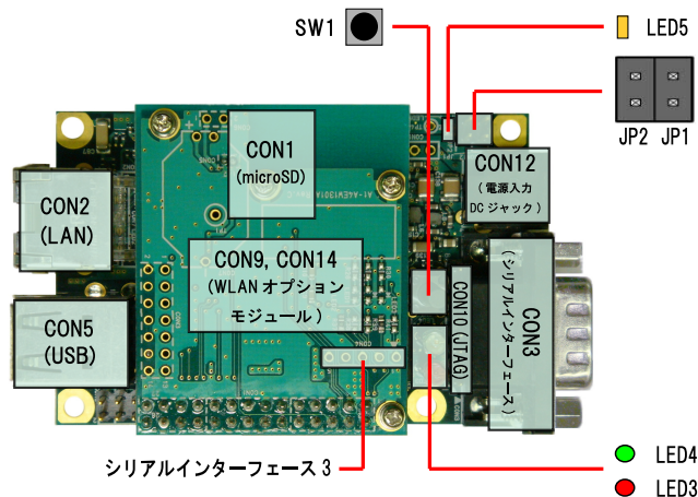
図 3.6 Armadillo-420 WLAN モデル見取り図
