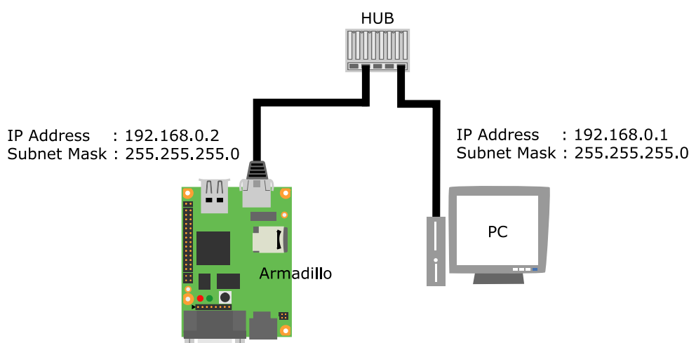
図 4.23 ネットワーク構成例
