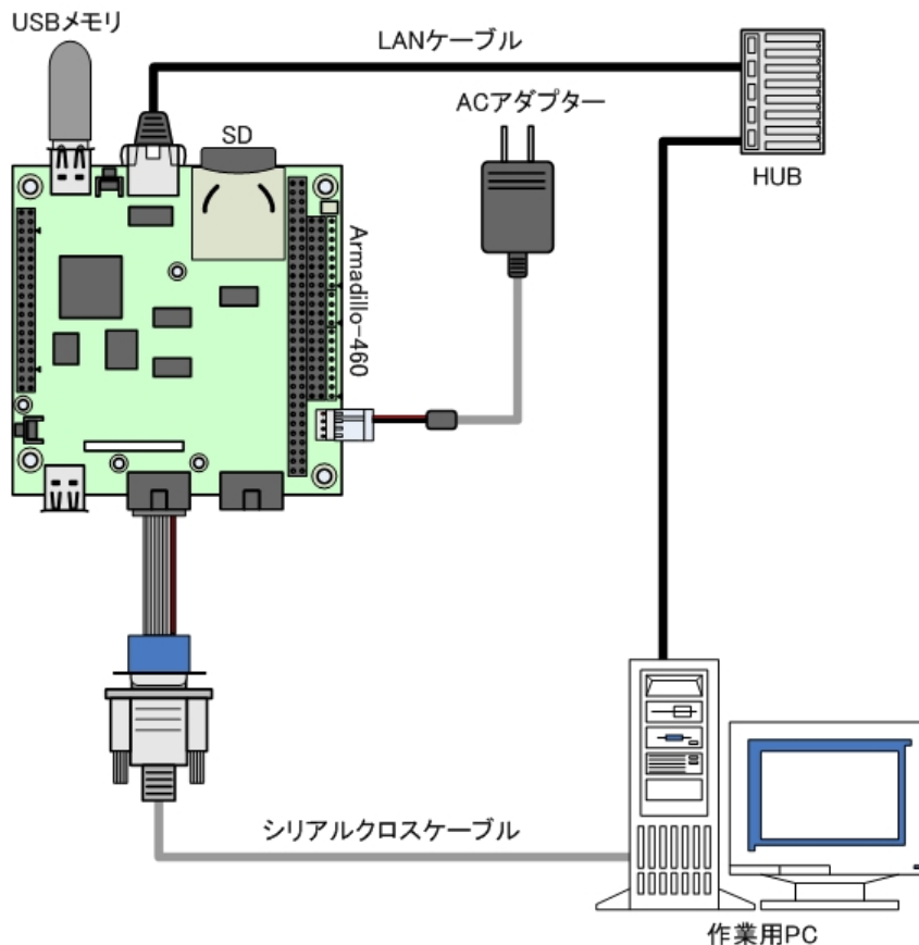
図 3.2 接続図
