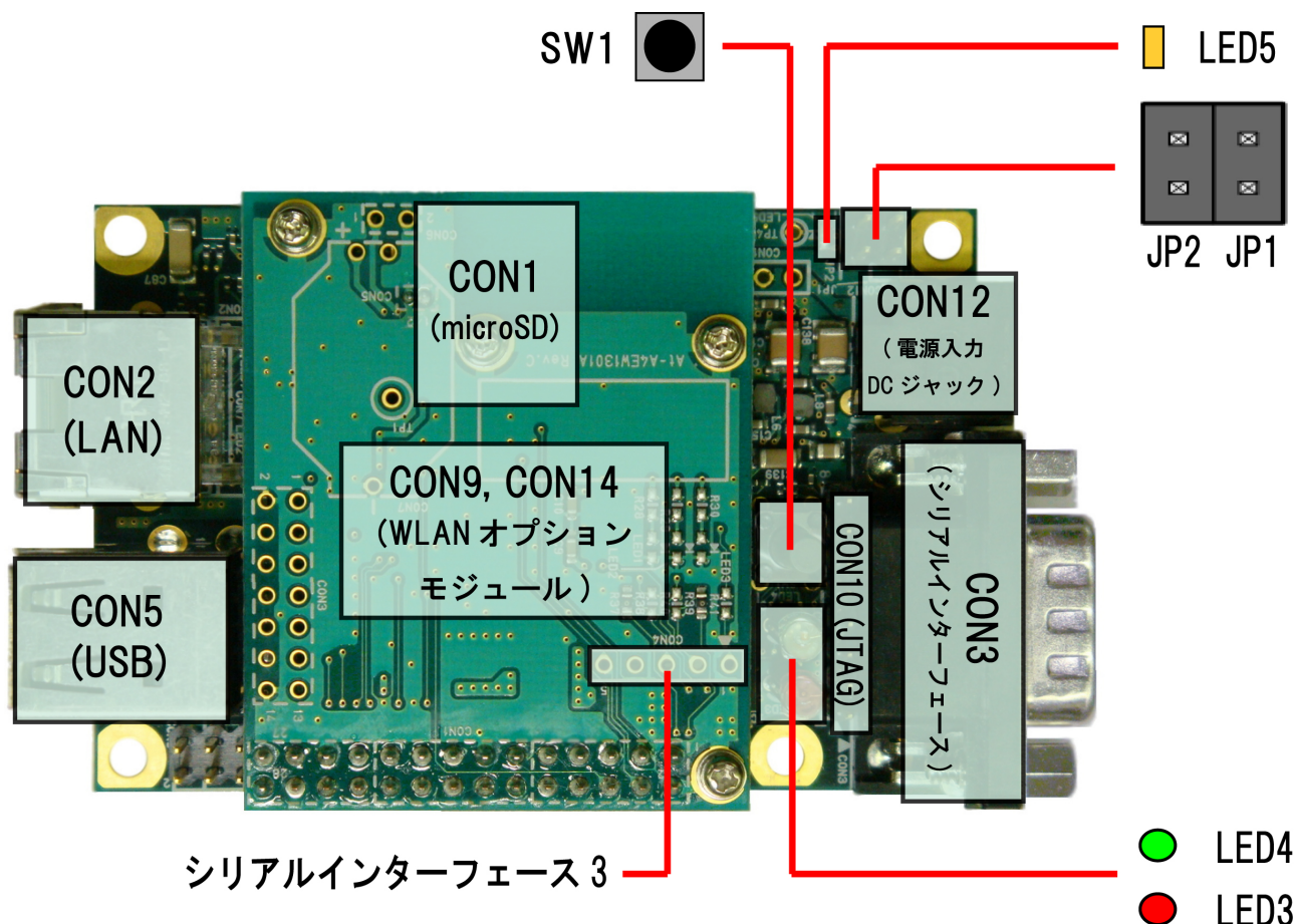
図 3.1 見取り図
