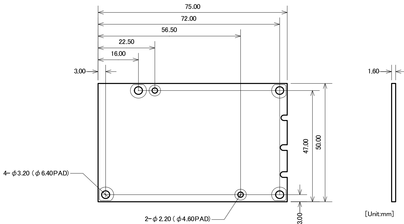
図 7.1 Armadillo-420 の基板形状および固定穴寸法
