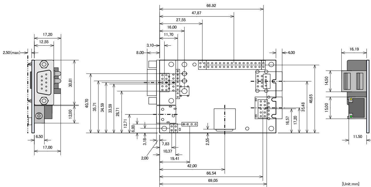
図 7.2 Armadillo-420 のコネクタ中心寸法
