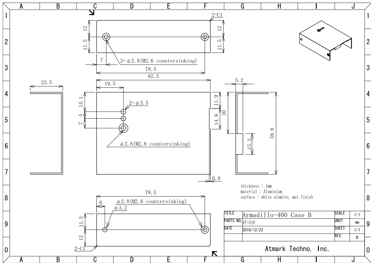
図 9.2 金属ケース(上板)寸法図
