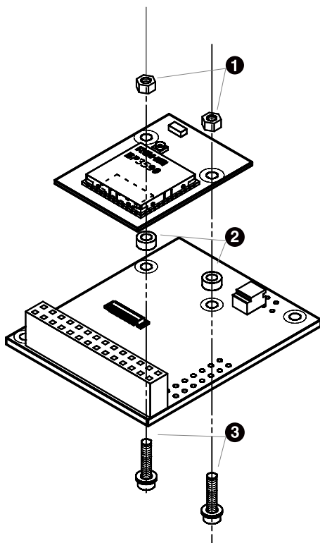
図 8.17 Armadillo-WLAN モジュールと WLAN インターフェースボードの組み立て図
