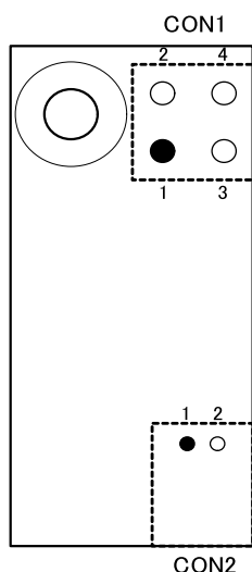
図 8.12 RTC オプションモジュール(型番：OP-A400RTCMOD-01)のインターフェース配置
