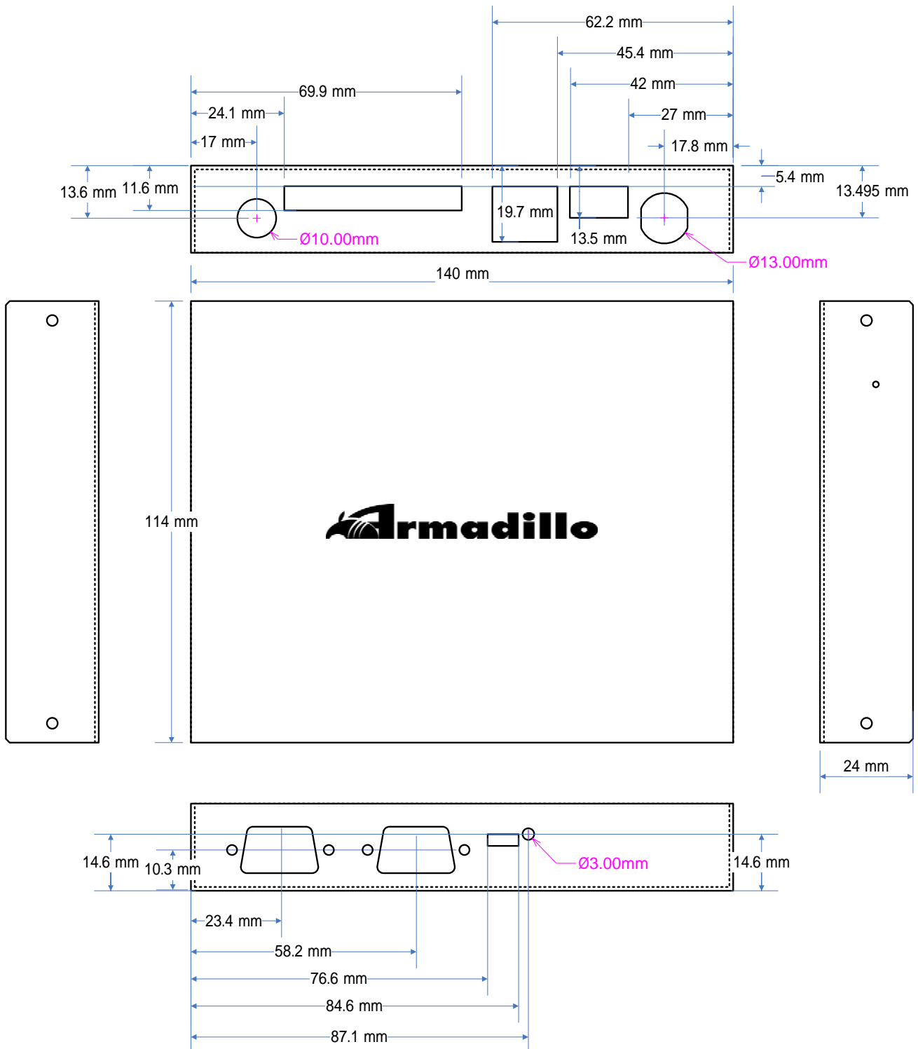
Armadillo-300 ケース形状図
