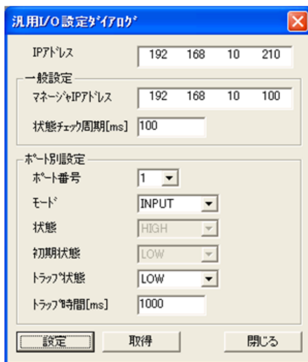
図 6.5 汎用 I/O の設定例
